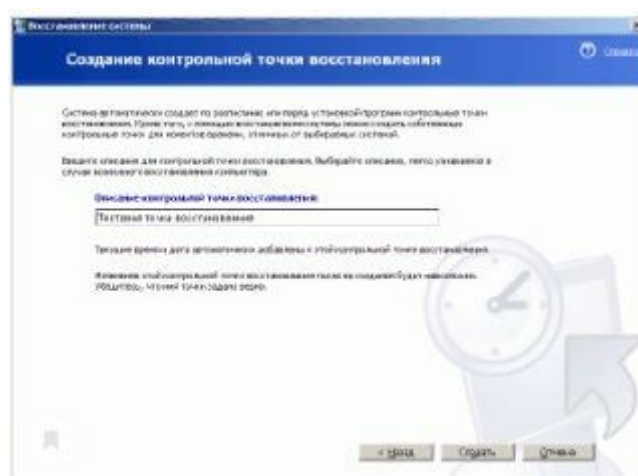
Восстановление системы.
