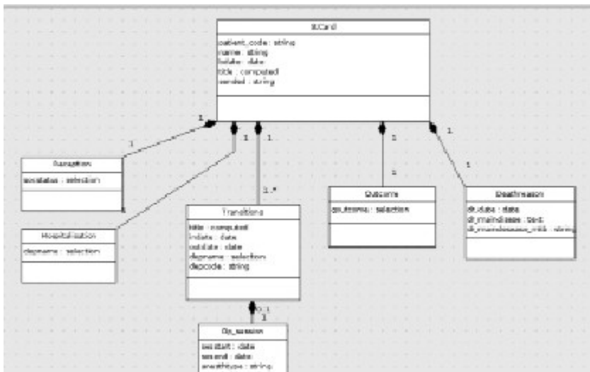
Рис. 1. Диаграмма классов
