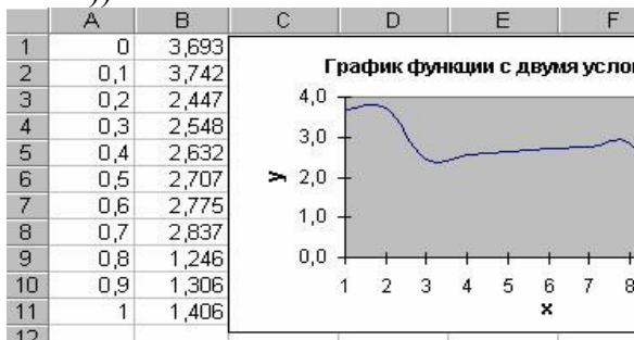
Рис. 3. График функции с двумя условиями
