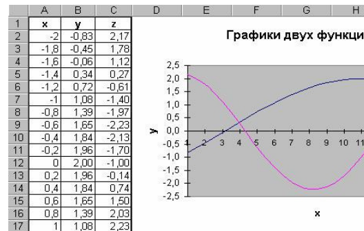
Рис. 4. График двух функций
